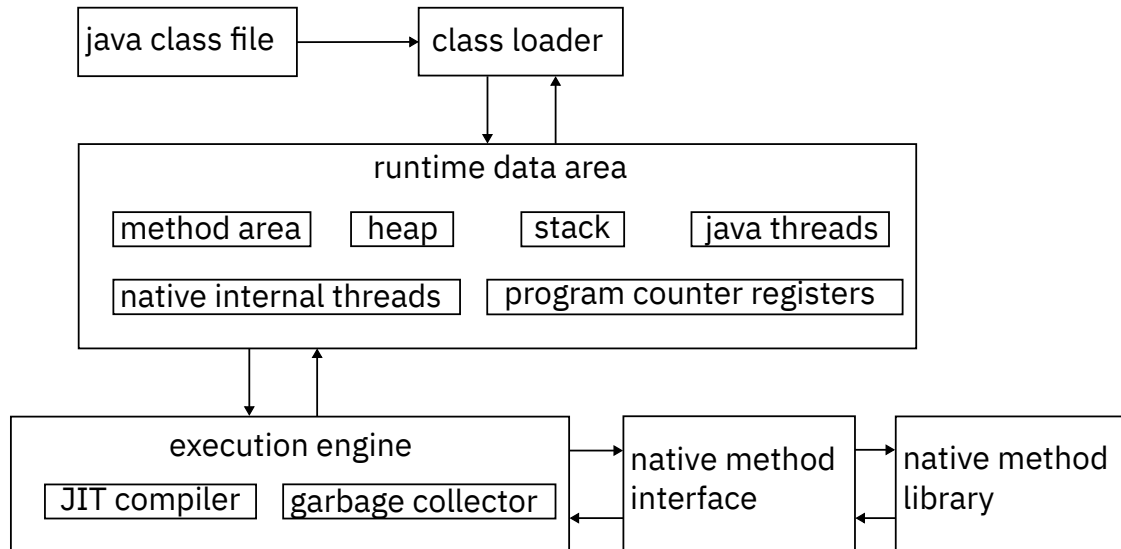
Рис. 1.2: Принцип работы JVM
