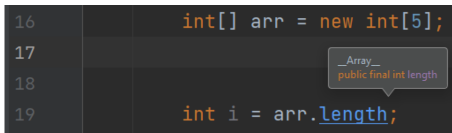
Рис. 1.13: Константа с длиной массива
