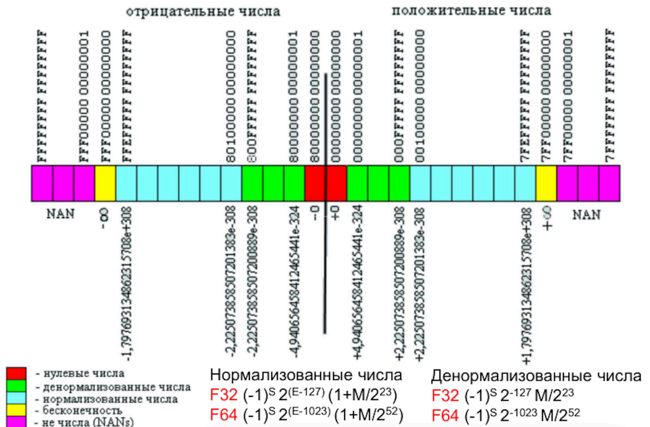
Рис. 5: Особенности работы с числами с плавающей запятой
